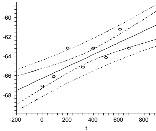
Figuur 24: Betrouwbaarheidsintervallen voor de y -waarden.
