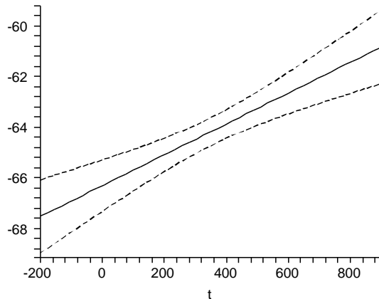
Figuur 23: Betrouwbaarheidsintervallen voor de gemiddelden \mu_x .
