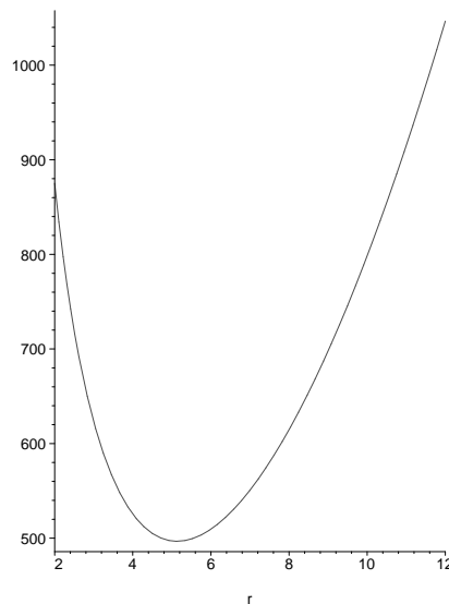
Figuur A.20: Oppervlakte van een blik van 850ml afhankelijk van de straal van het grondvlak
