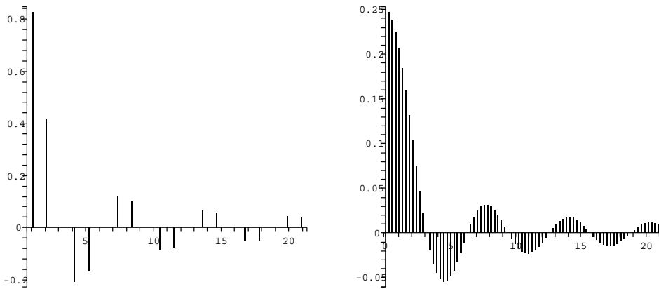
Figuur I.18: Fourier coëfficiënten voor rechthoek impuls met periode L en 4L .
