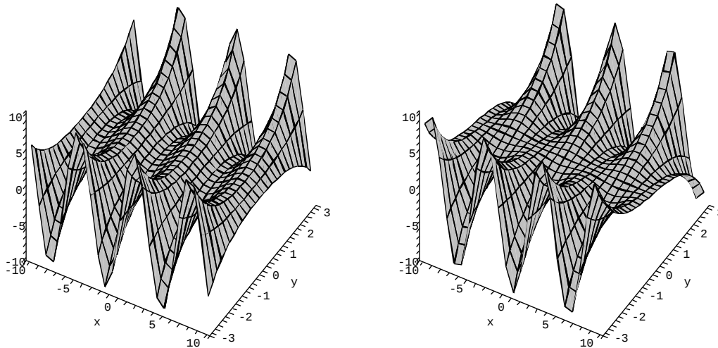
Figuur I.25: Reëel en imaginair deel van \sin(z)
