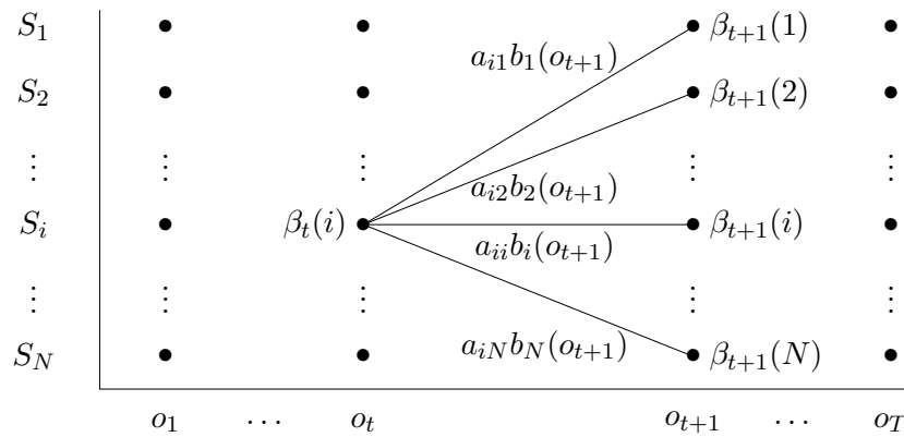
Figuur III.6: Berekening van \beta_t(i) in het backward algoritme .
