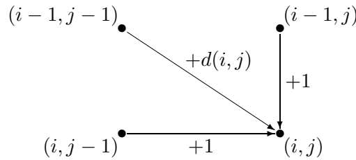
Figuur III.9: Mogelijke voorgangers van (i, j) .
