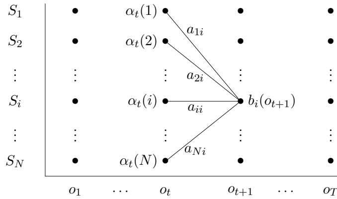
Figuur III.5: Berekening van \alpha_{t+1}(i) in het forward algoritme .
