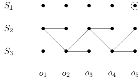
Figuur III.8: Tralie voor het Viterbi algoritme.
