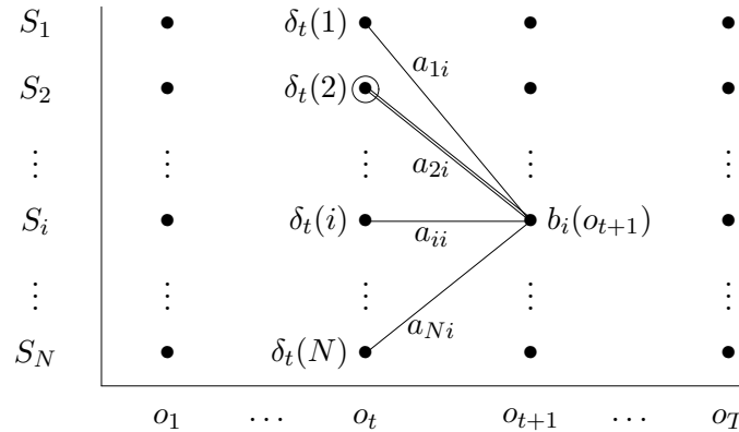
Figuur III.7: Berekening van \delta_{t+1}(i) in het Viterbi algoritme.
