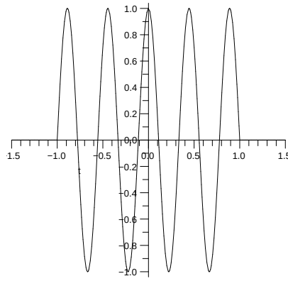
Figuur II.16: Eindige cosinus golf tussen t = -1 en t = 1 .
