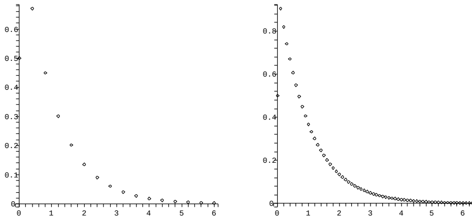
Figuur II.30: Discretisering van een exponentiële daling met 16 (links) en 64 punten (rechts).
