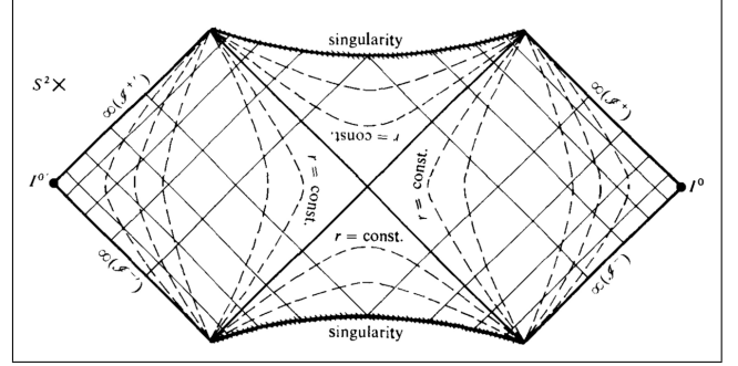
Penrose diagram van Kruskal ruimte-tijd [22, p. 208, Fig. 37].
